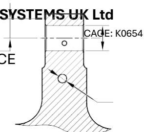
СЕЧЕНИЕ С-С ОТВЕРСТИЕ ЗВЕНА ФИКСАТОРА
